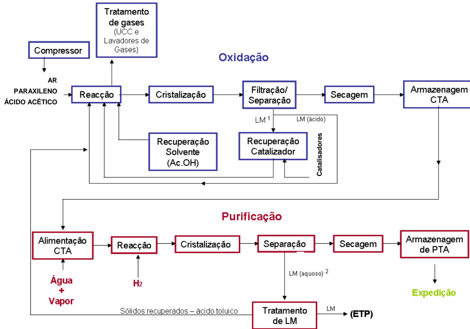
Figura 1 – Diagrama de Processos (LM – Licor Mãe; UCC – Unidade de Combustão Catalítica)
